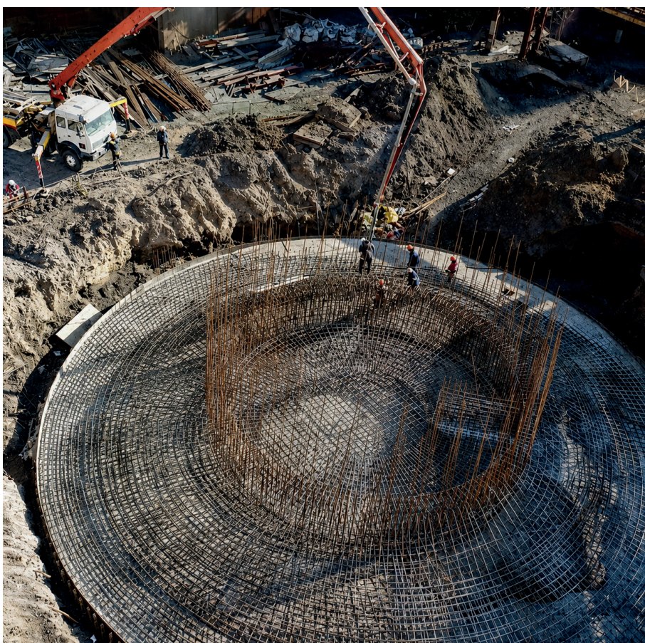
«Строительство дымовой трубы Н=150м, ТЭЦ-ПВС» АО «АрселорМиттал Темиртау»
